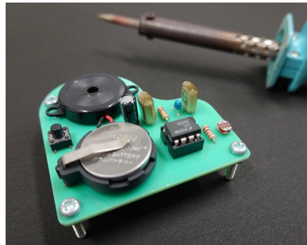
▲ 完成した電子楽器
