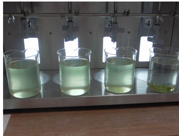
薬品を使った水処理実験
