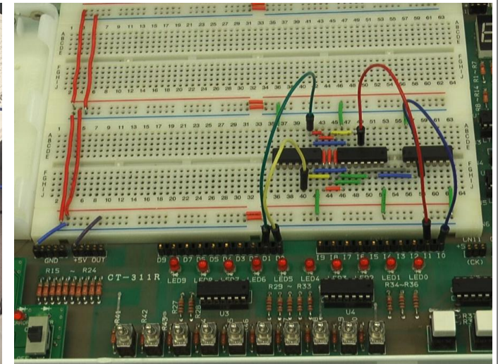
製作した回路の例
