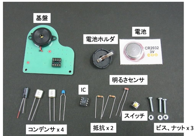
▲ 製作に使う部品
