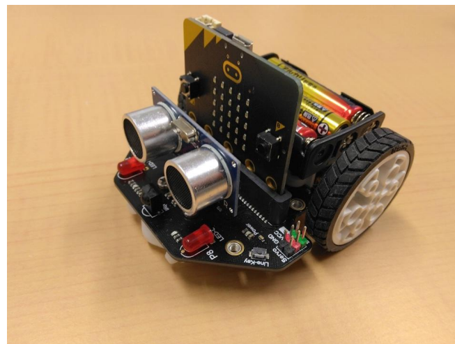
▲ ロボットカー
