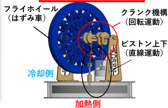
3Dモデル (シミュレーション)
